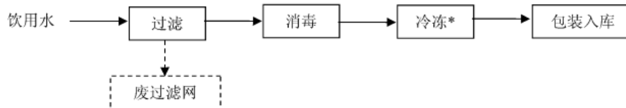
食用冰生产工艺流程及产污环节图
